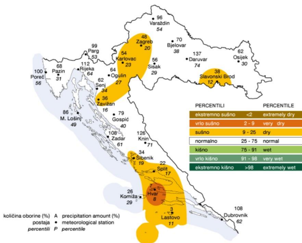
Slika 5. Odstupanje količine oborine za Republiku Hrvatsku, kolovoz 2018. godine
