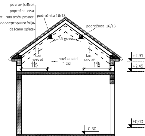
PRESJEK B-B M 1:100
