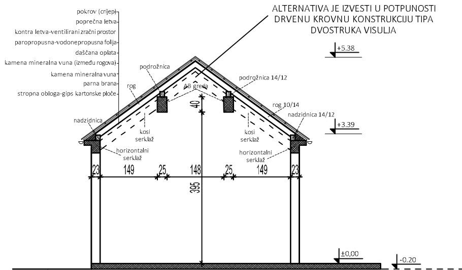
PRESJEK A-A M 1:100
