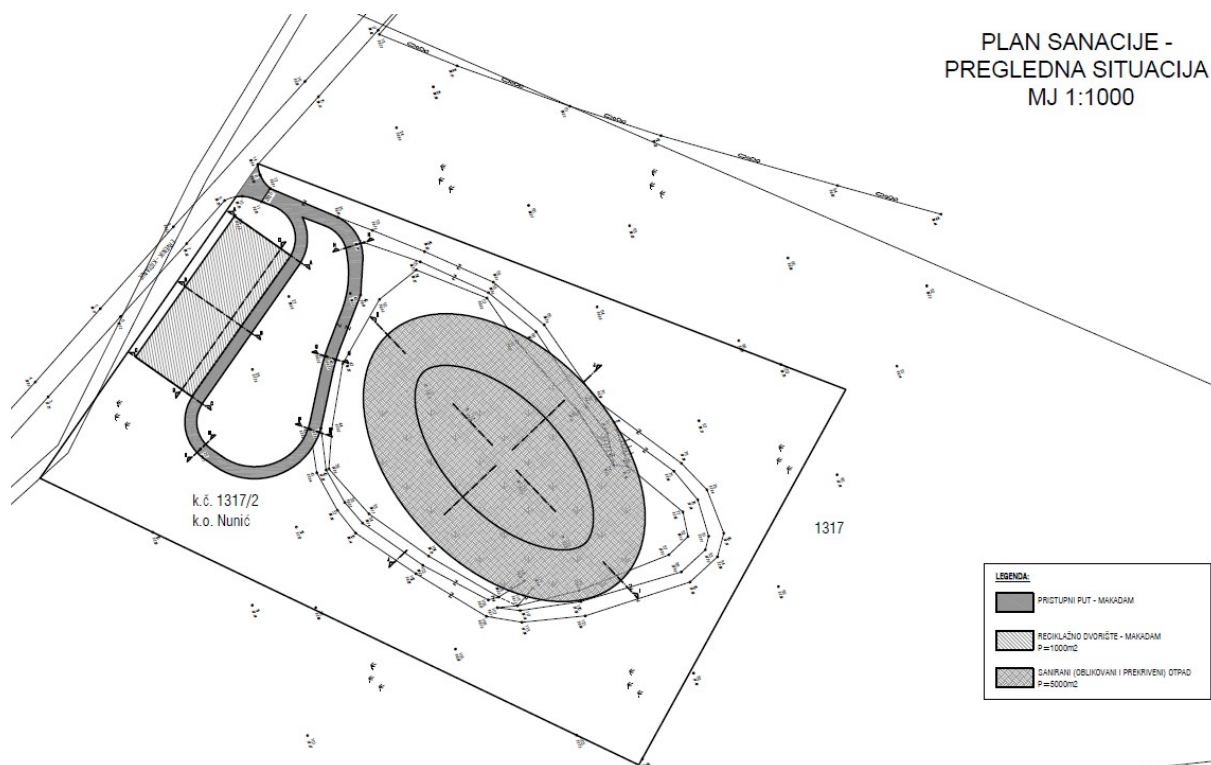
Slika 3: Situacija – plan sanacije odlagališta
